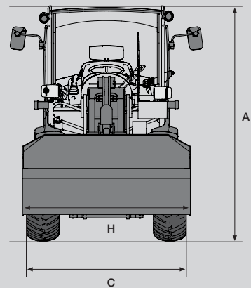
Mit Standardschaufel und Standardbereifung (Frontansicht)
